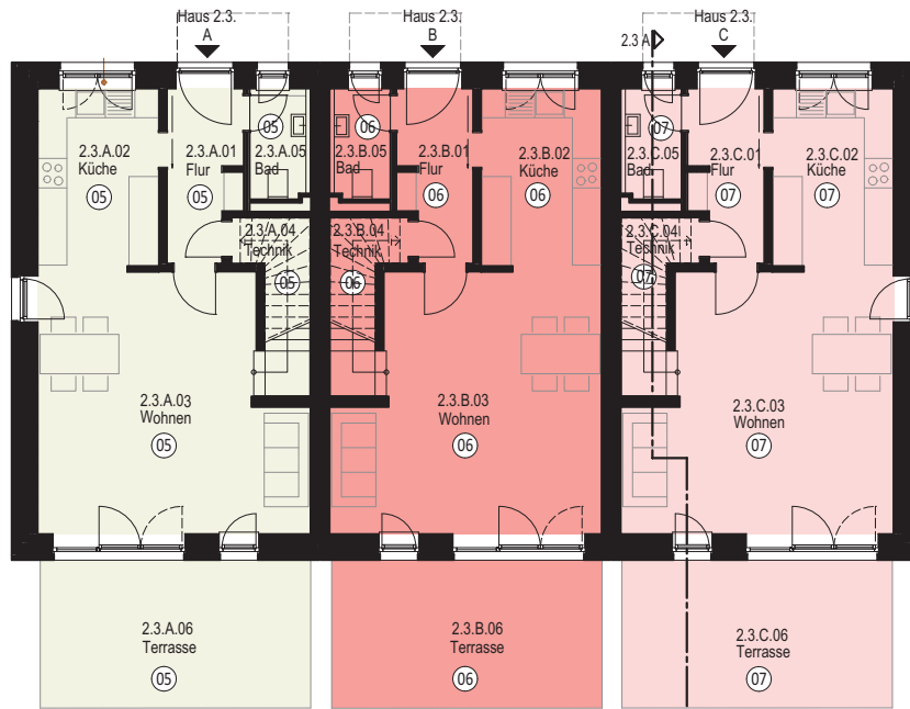
ERDGESCHOSS
