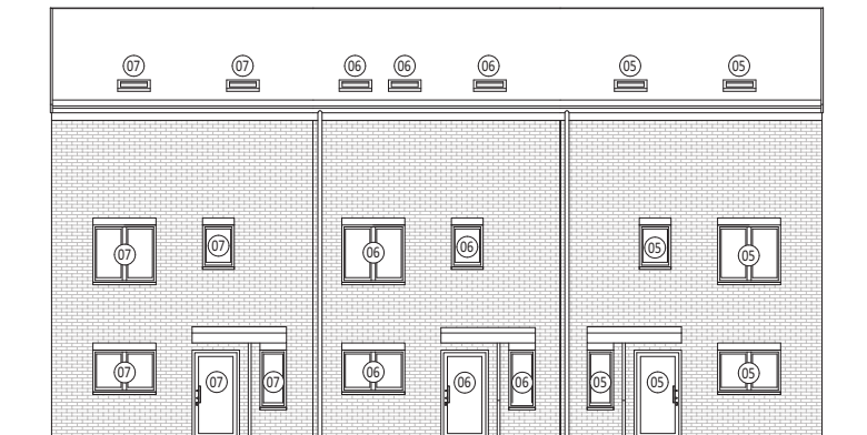
ANSICHT OST
