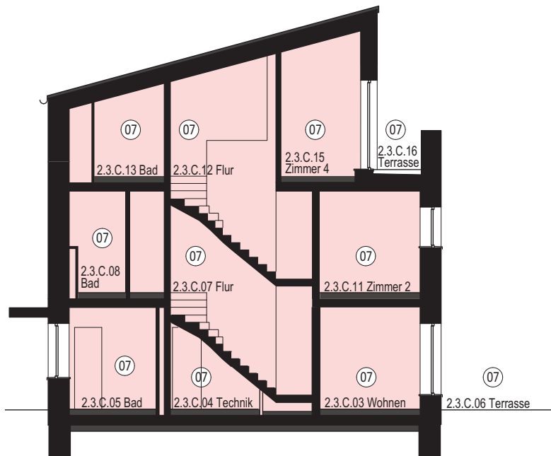
SCHNITT
