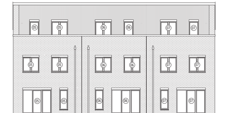
ANSICHT WEST
